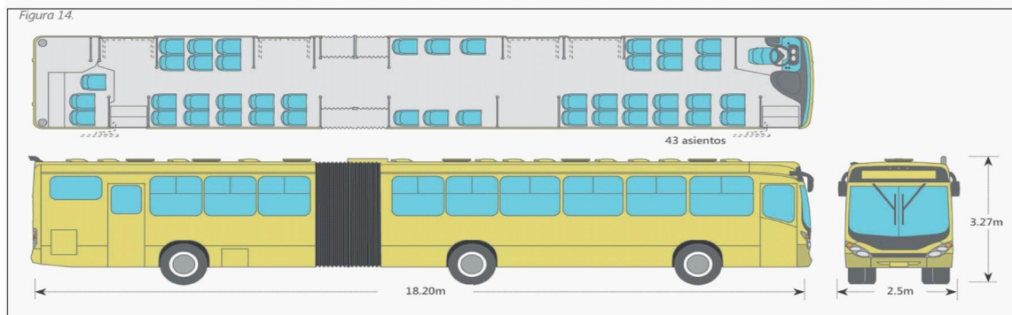
Figura 13. Dimensiones bus urbano Figura 14. Dimensiones autobús articulado Fuente: Elaboración propia
