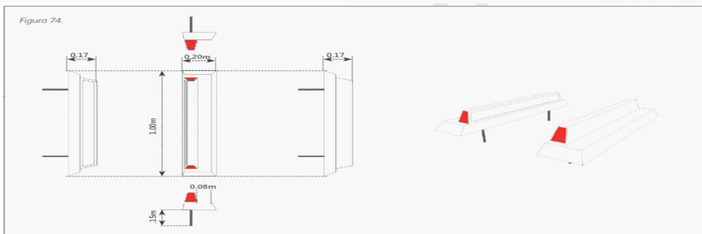
Barra de confinamiento Tipo "L"
