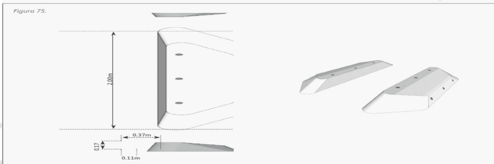
Barra de confinamiento Tipo "Trapezoidal"
