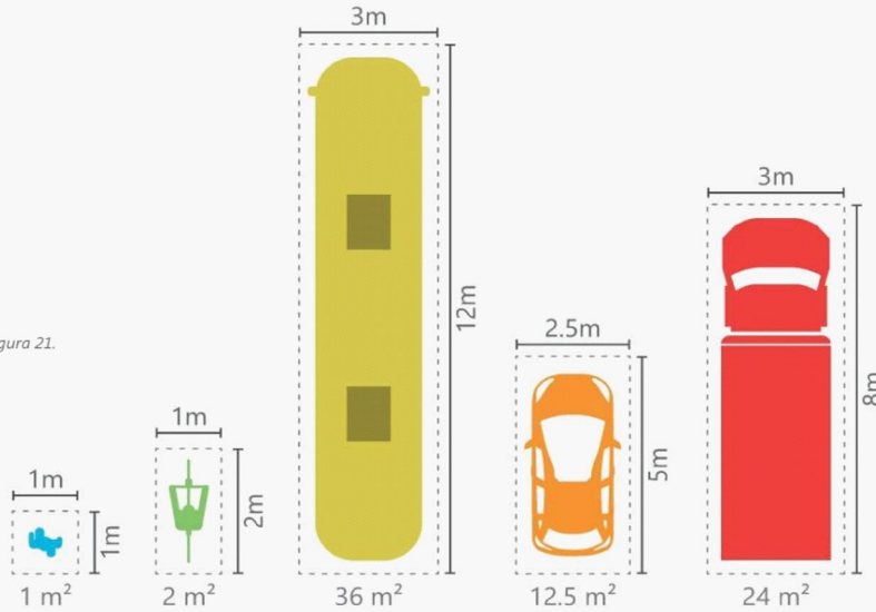
Figura 21. Dimensiones y velocidades de los diferentes medios de transporte Fuente: (NACTO, Global Street Design Guide, 2016)
